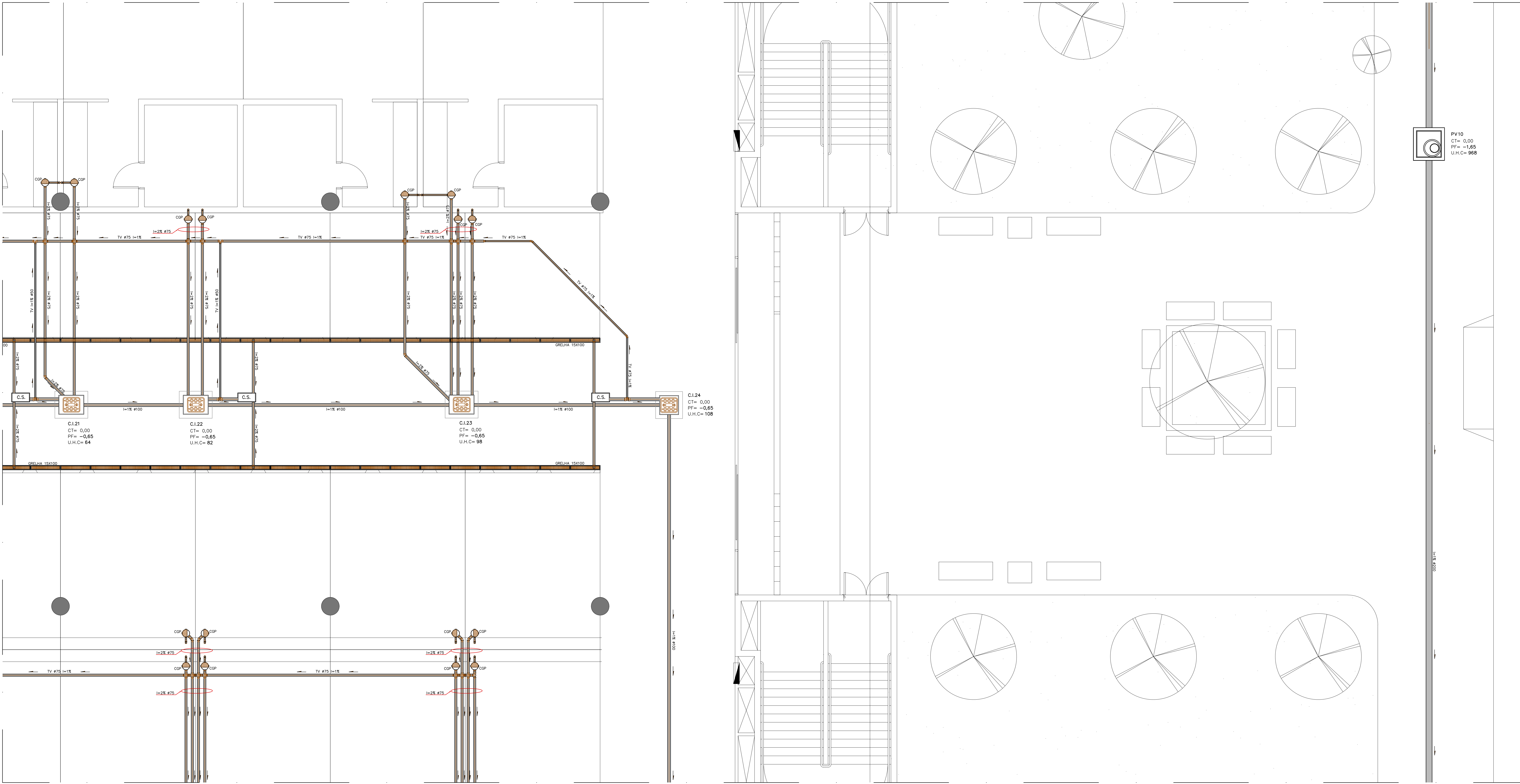
TÉRREO ESGOTAMENTO SANITÁRIO - JUNTA "N" ESC.:1/50
