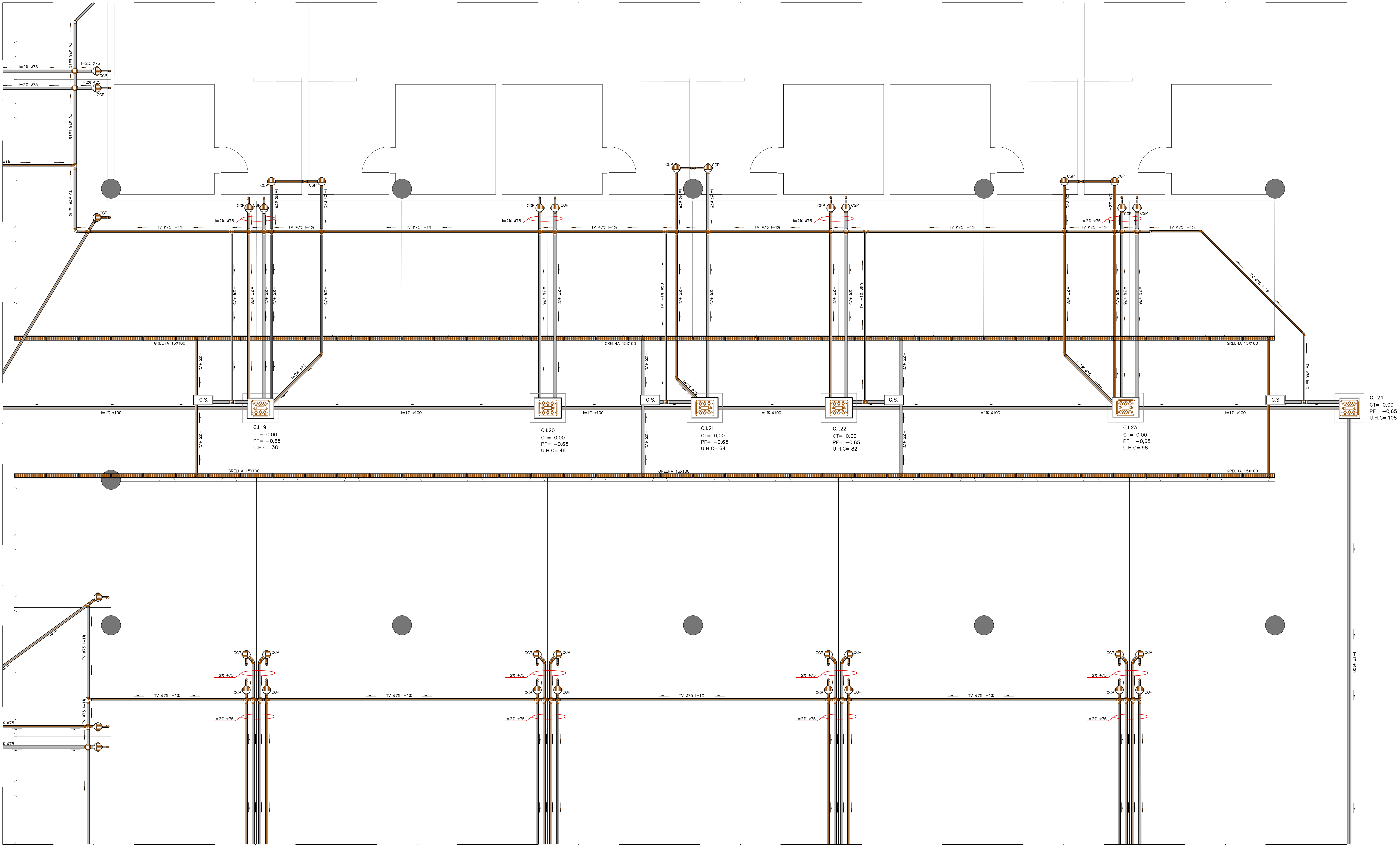
TÉRREO ESGOTAMENTO SANITÁRIO - JUNTA "K" ESC.:1/50
