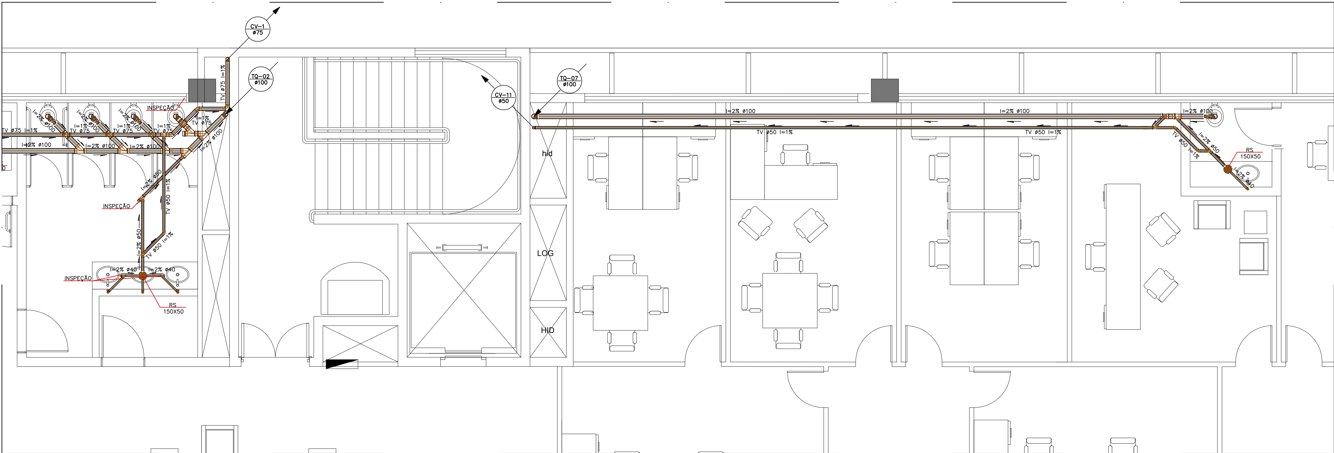
2º PAVIMENTO ESGOTAMENTO SANITÁRIO - JUNTA "B" ESC.:1/50
