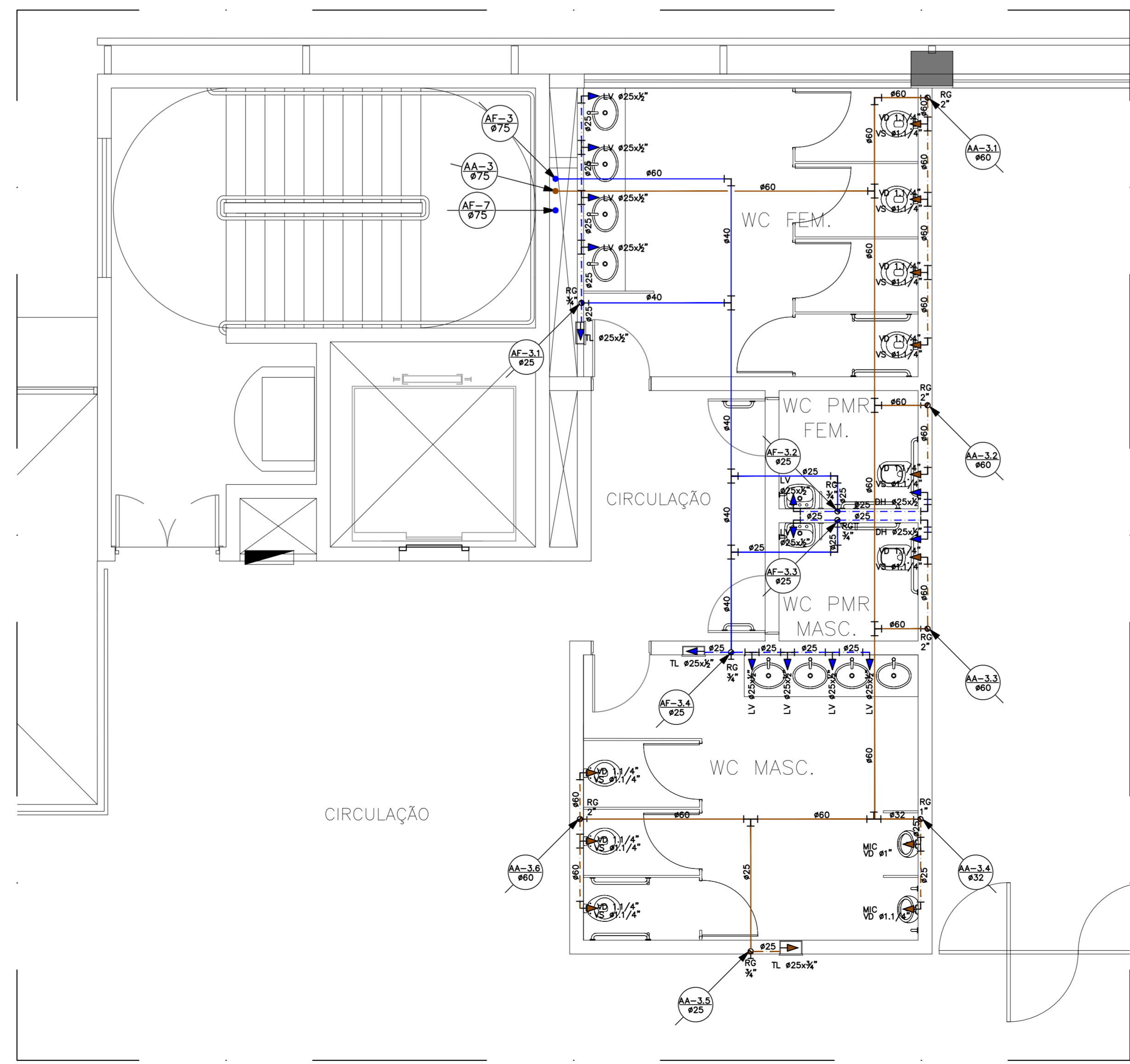
1º PAVIMENTO ÁGUA FRIA/APROVEITAMENTO - JUNTA "C" ESC.:1/50
