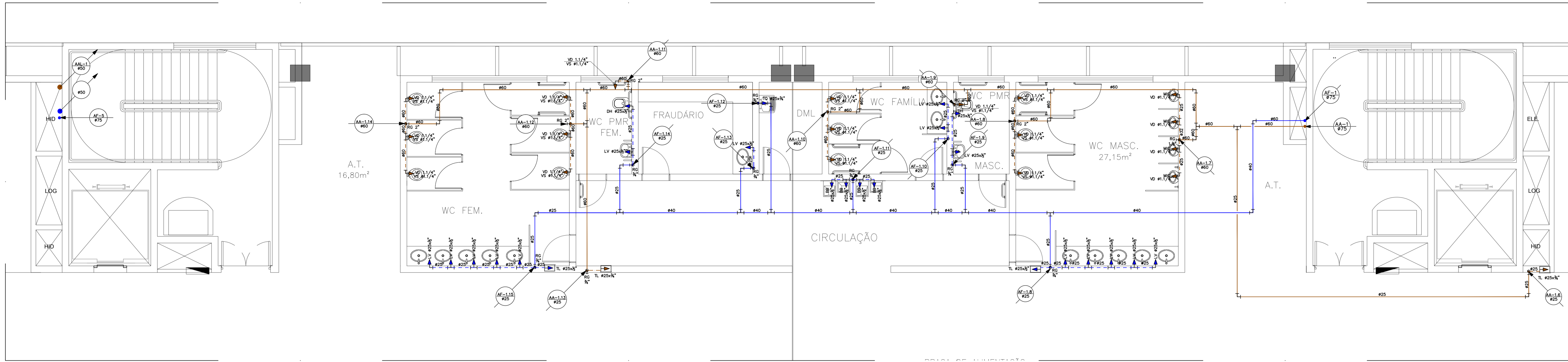
1º PAVIMENTO ÁGUA FRIA/APROVEITAMENTO - JUNTA "A" ESC.:1/50
