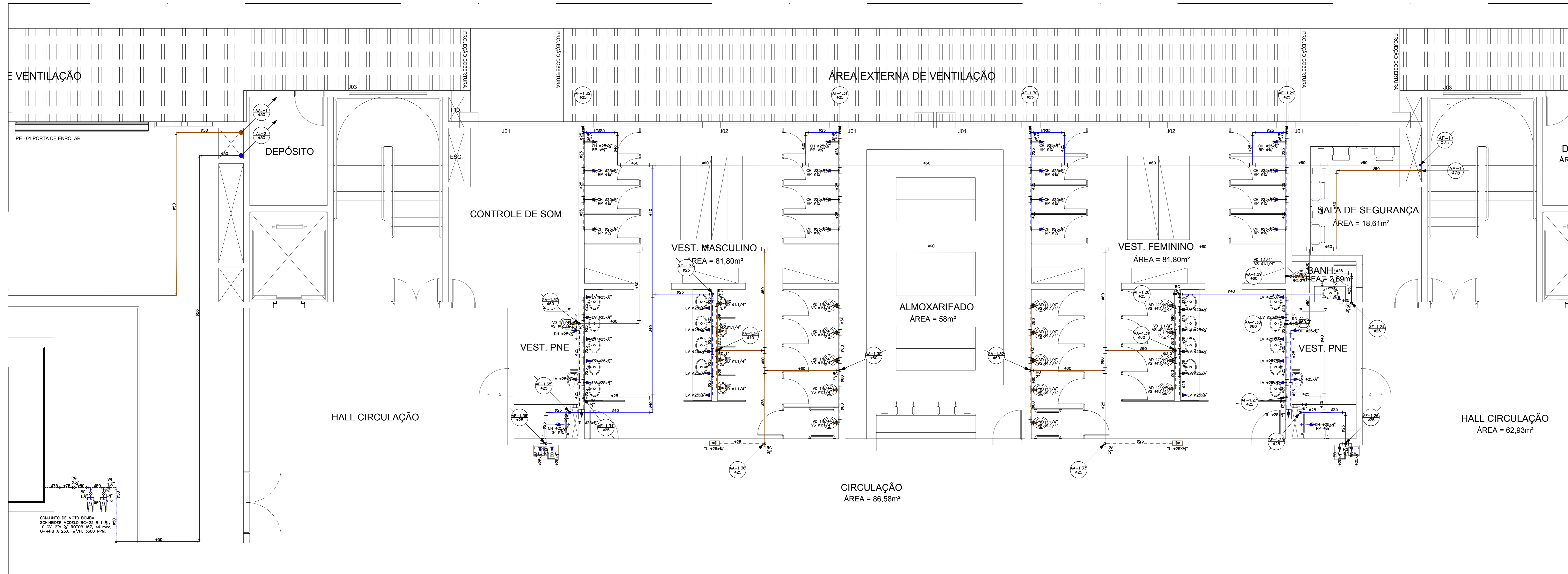
SUBSOLO ÁGUA FRIA/APROVEITAMENTO - JUNTA "A" ESC.:1/50
