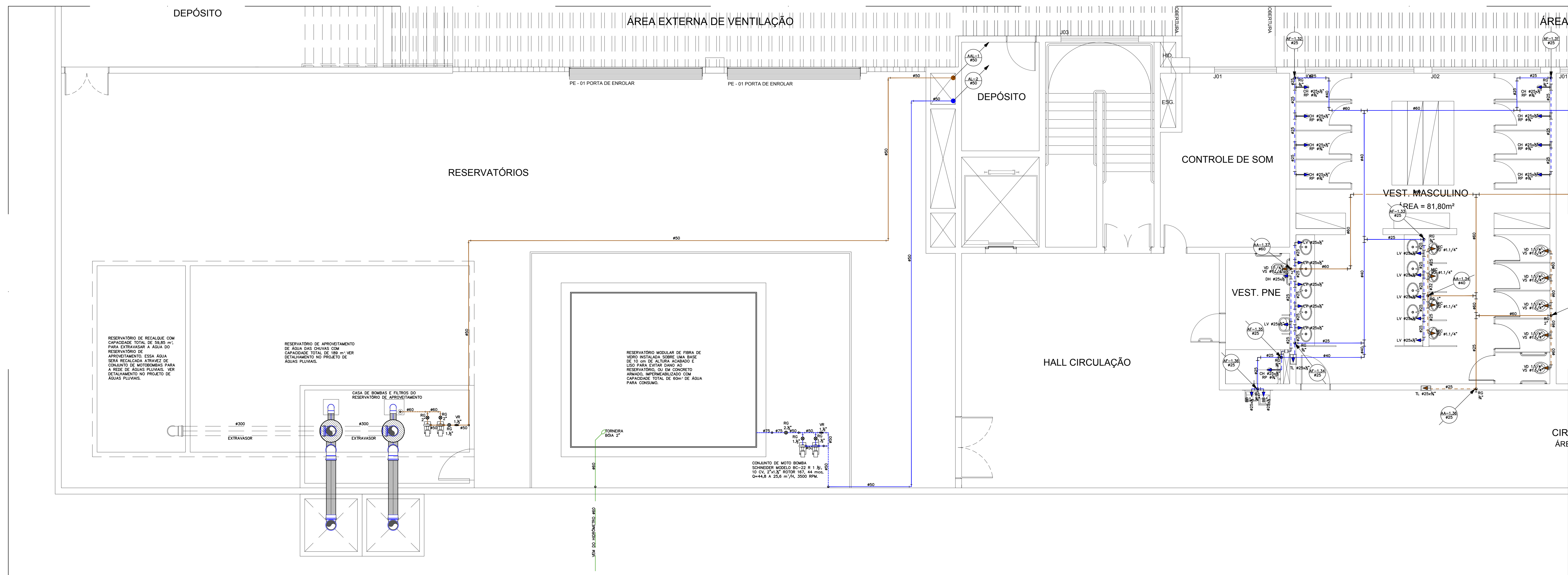
SUBSOLO ÁGUA FRIA/APROVEITAMENTO - JUNTA "B" ESC.:1/50
