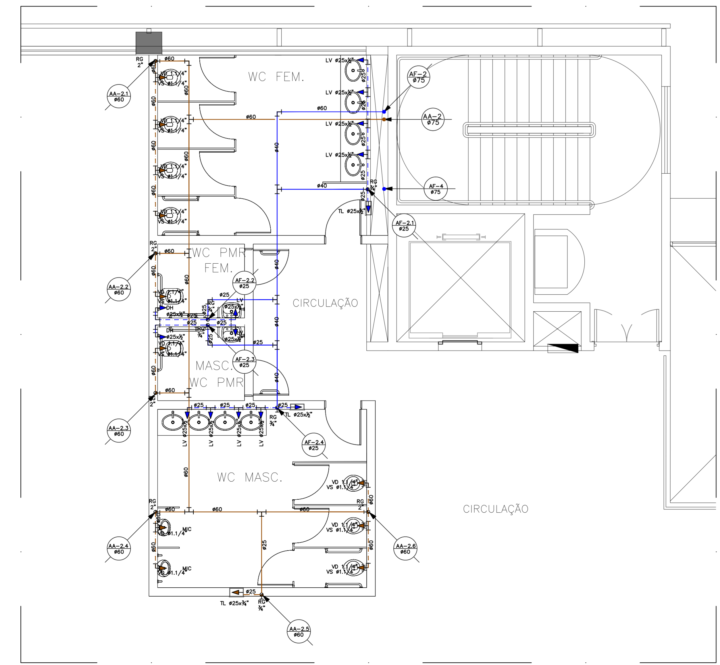
1º PAVIMENTO ÁGUA FRIA/APROVEITAMENTO - JUNTA "B" ESC.:1/50
